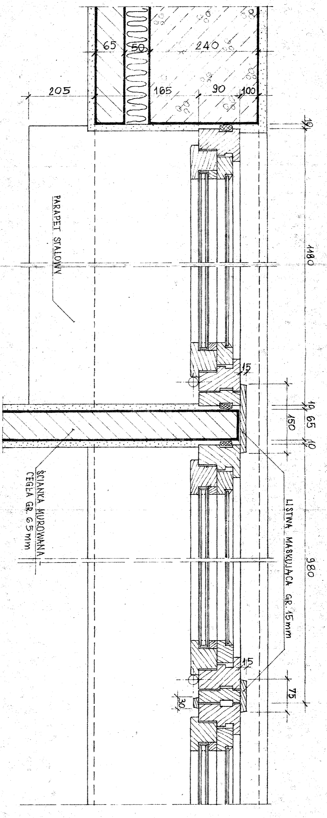
OKNA ZESPOLONE ZE ŚCIANKĄ MUROWANĄ GRUB 65mm SKALA 1:5
