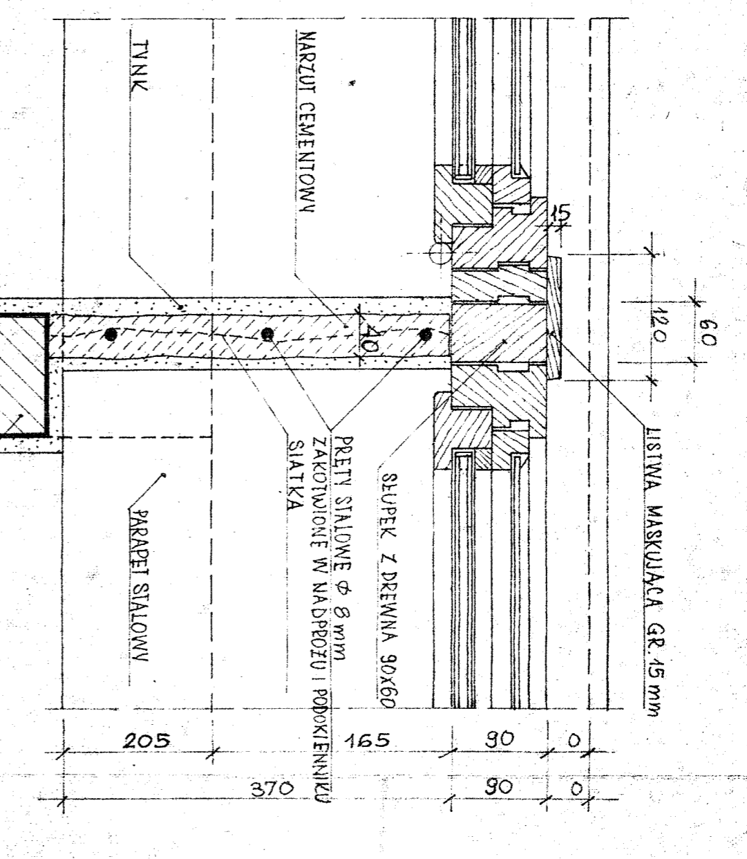
OKNA ZESP. Z TYNKIEM NA SIATCE 1:5
