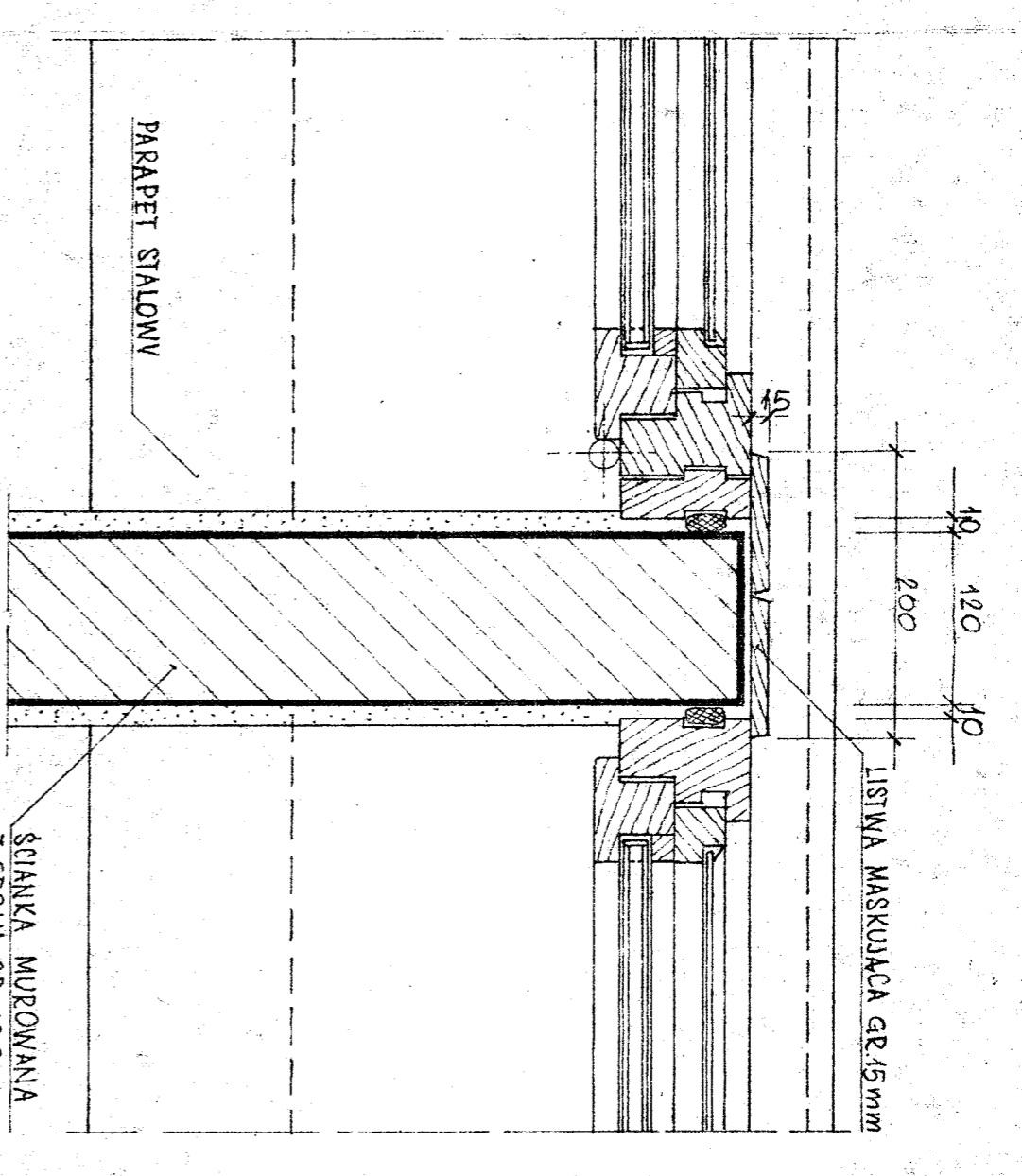
OKNA ZESP. ZE ŚCIANKĄ GRUB 120mm
